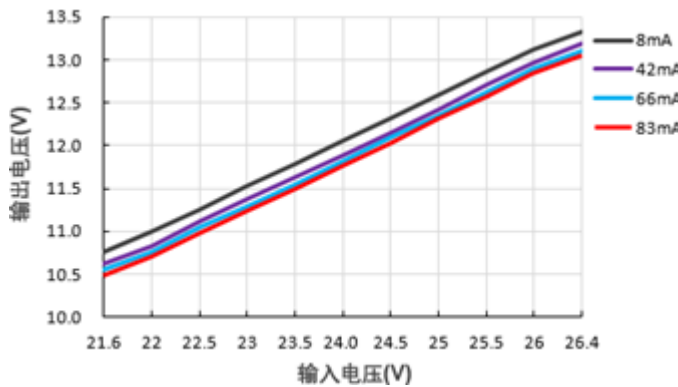
输出电压Vs输入电压 (PS01-F24SC24)
