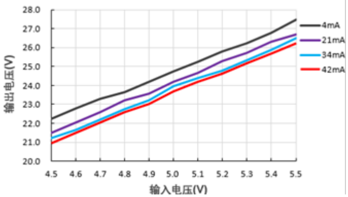
输出电压Vs输入电压 (PS01-F12SC05)
