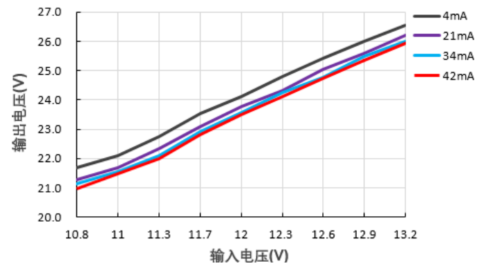
输出电压Vs输入电压 (PS01-F12SC24)
