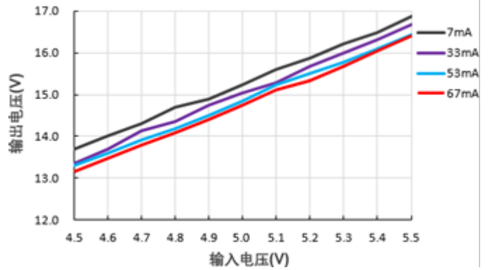
输出电压Vs输入电压 (PS01-F12SC03)
